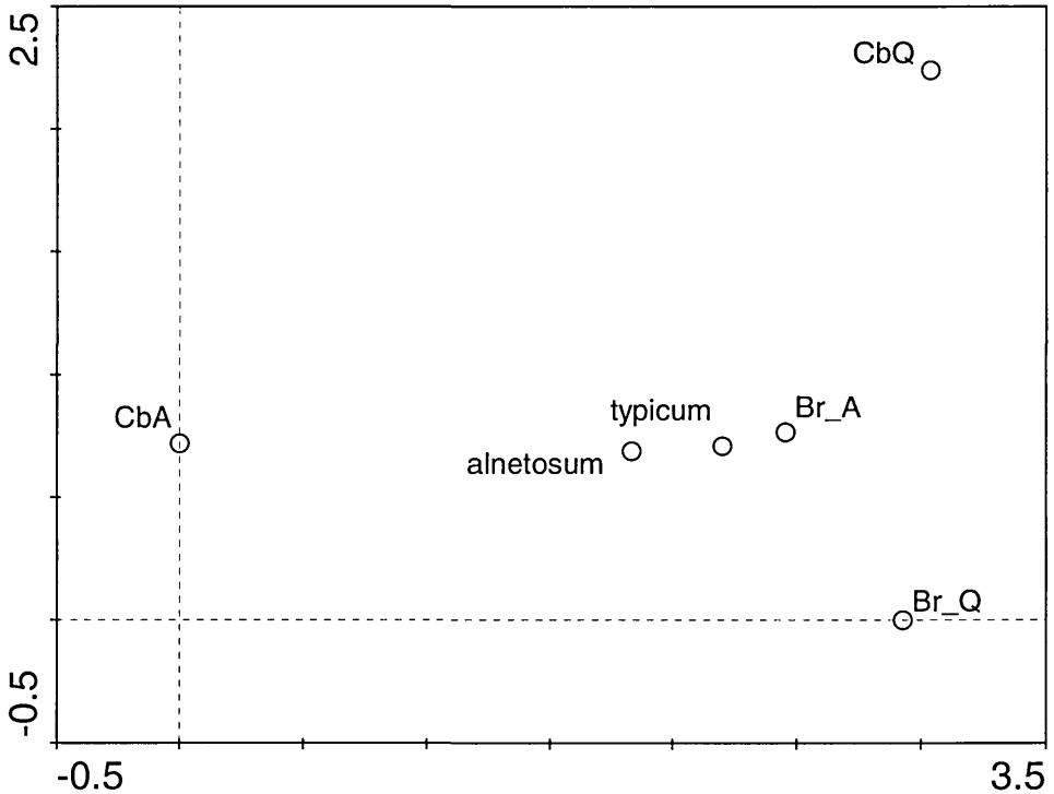
Abb.3. Ähnlichkeit der Auenwald-Einheiten nach dem DCA-Biplot-Schaubild ( \lambda_1 = 0,52 ; \lambda_2 = 0,31 , die ersten zwei Achsen zeigen 47% der Variabilität). – Similarity of alluvial forest units according to the DCA-Biplot.
