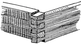
Ściana zrębowa
