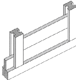
Ściana sumikowo-łątkowa
