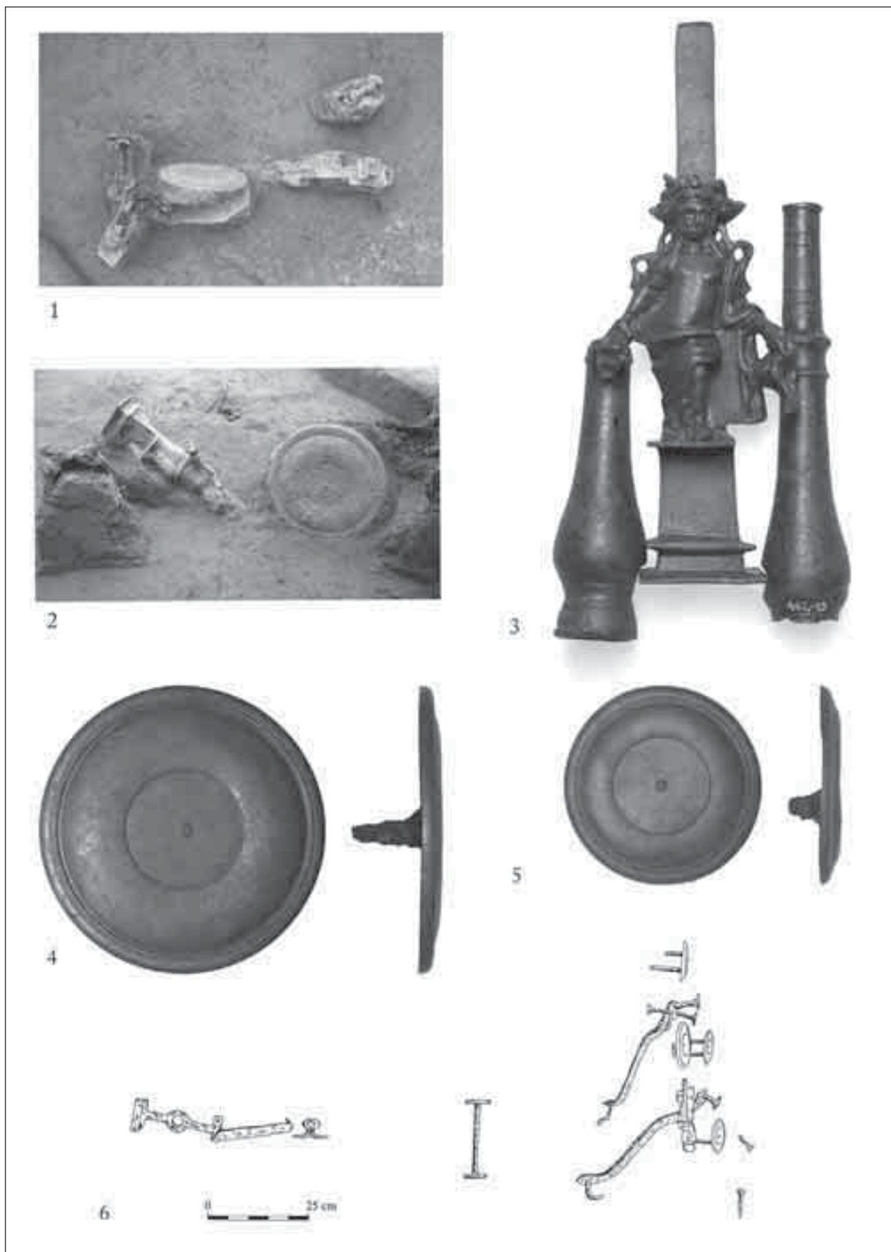
10. kép: 162. kocsisír. 1–2: a hátsó vánkös bronzdíszítményei feltárásuk helyzetében; 3: Bacchus bronzszobra; 4–5: a nagy- és kiskorongok a hátsó vánkös hátsó oldaláról; 6: a nyújtó- és a vánkös alkatrészei (rajz: Mráv Zsolt)
