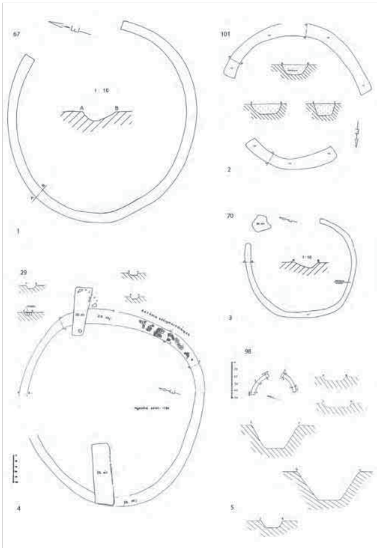
77. kép: Körárkok: 67, 101, 70, 29, 98. árok metszetei
