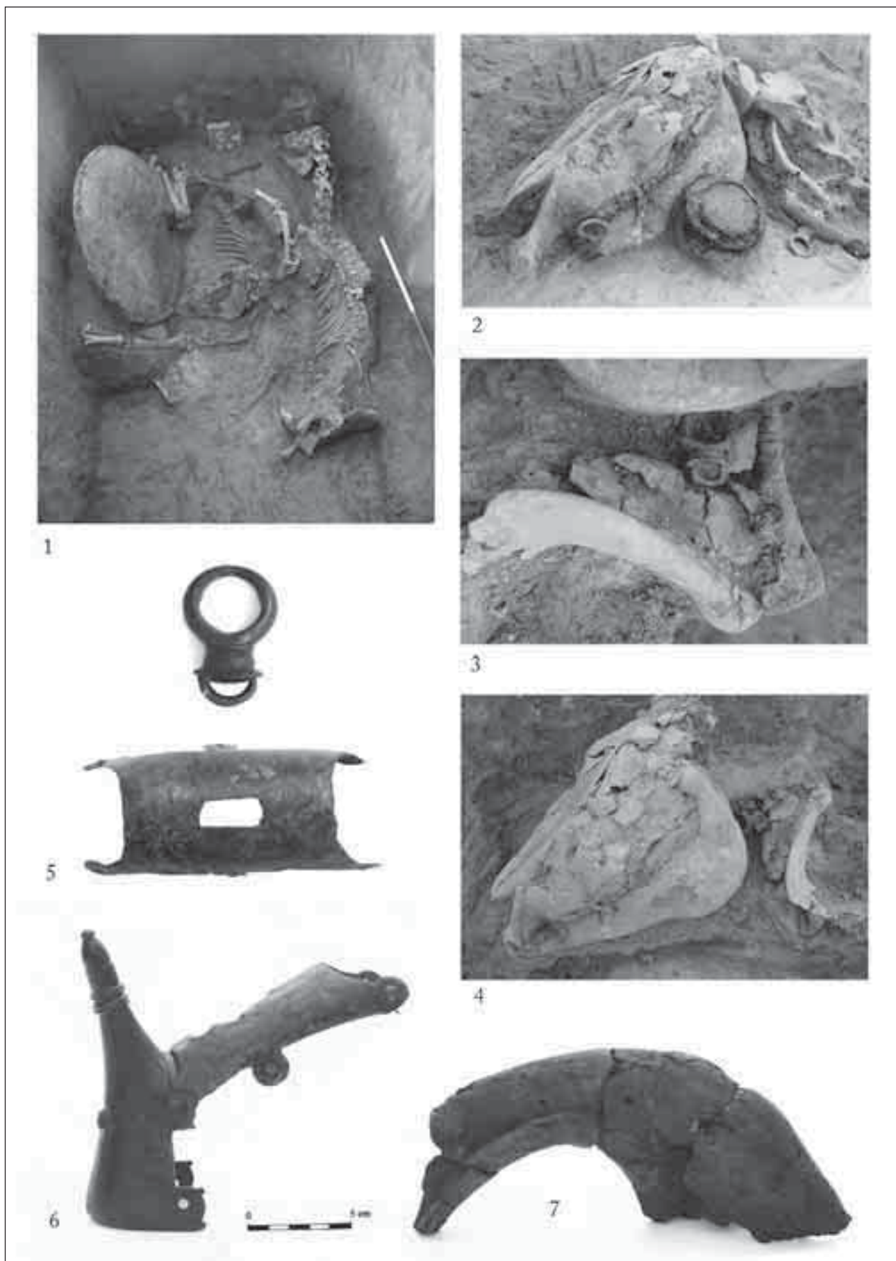
6. kép: 124. kocsisír. 1: a két fogatos ló váza a sírgödör alján; 2–4: az 1. ló jármának veretei feltárásuk pozíciójában; 5–7: és restaurálásuk után
