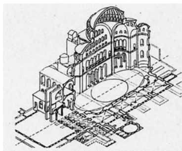
Hagia Szophia térmetszete
