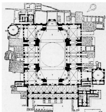
Hagia Szophia alaprajza
